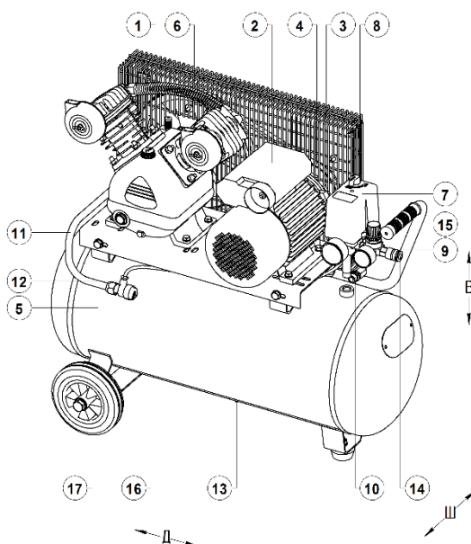
Рисунок 4 - Общий вид компрессора СБ4/С-50.LB24А
