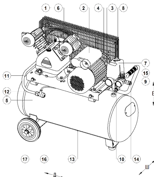
Рисунок 4 - Общий вид компрессора СБ4/С-50.LB24
