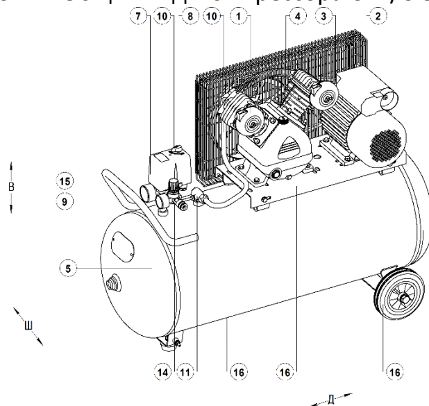
Рисунок 5 - Общий вид компрессора СБ4/С-100.LB24
